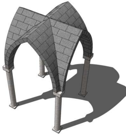
КРЕСТОВЫЙ СТРЕЛЬЧАТЫЙ СВОД
