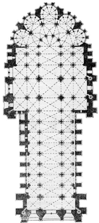
Собор в Реймсе. План
