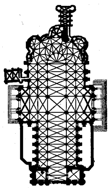
План Шартрского собора
