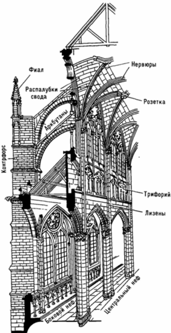
КРЕСТОВЫЙ СТРЕЛЬЧАТЫЙ СВОД
