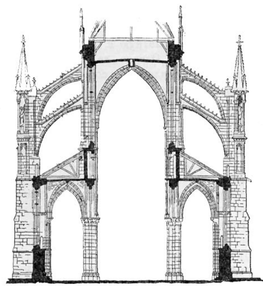
Собор в Реймсе, поперечный разрез
